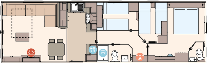
40FT X 12FT X 3 BEDROOM
