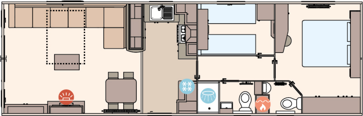
38FT X 12FT X 2 BEDROOM
