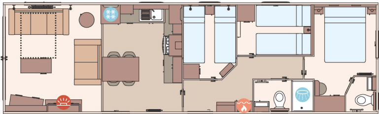
40FT X 12FT X 3 BEDROOM
