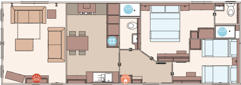
PREMIER 40FT X 14FT X 2 BEDROOM
